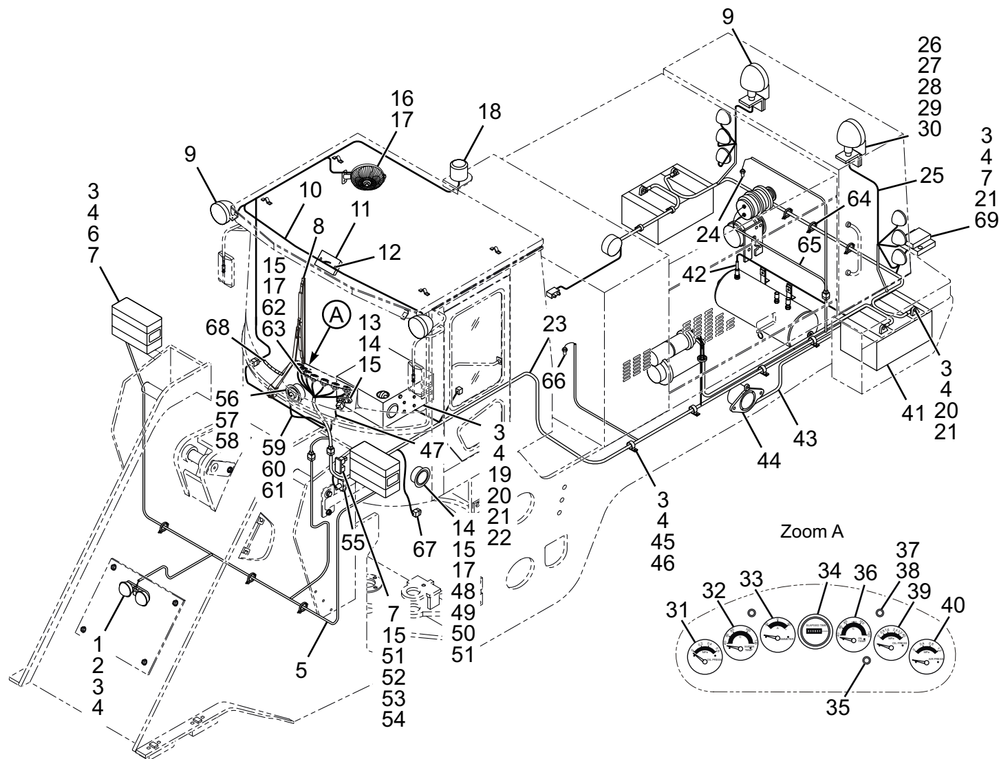
电器系统 Electrical System (CDM853.15 V) ( 图 /Figure 37)
