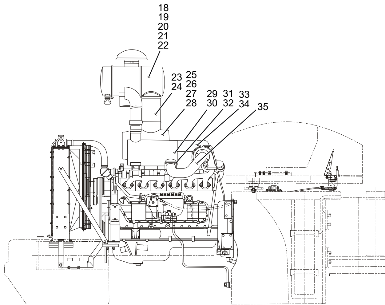
DH615G0430 柴油机系统 DH615G0430 Diesel Engine Assembly (CDM853.01)( 图 /Figure 01)
