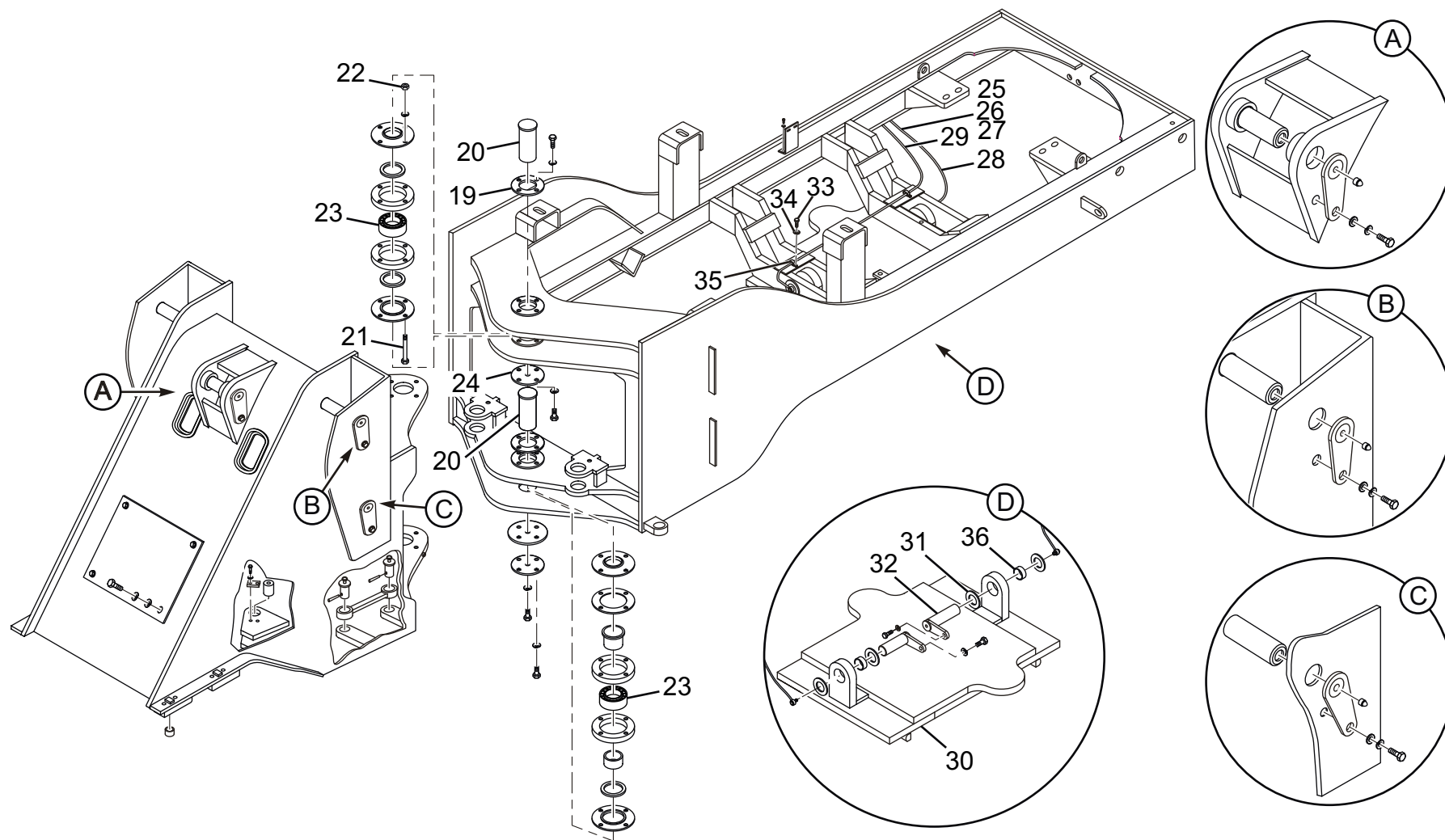
车架系统 Frame System (CDM853.10) ( 图 /Figure 33)
