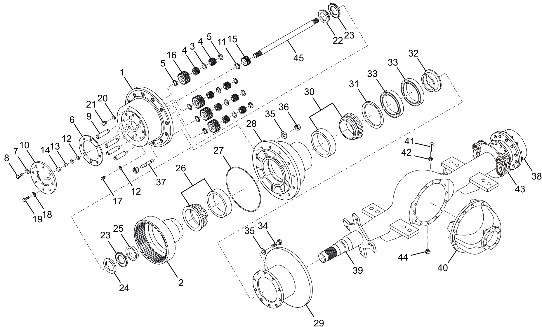
标准 50F 驱动桥 Standard 50F Axle II ( LG50F.04500A 前桥用 LG50F.04800A 后桥用 )( 图 /Figure 20)
