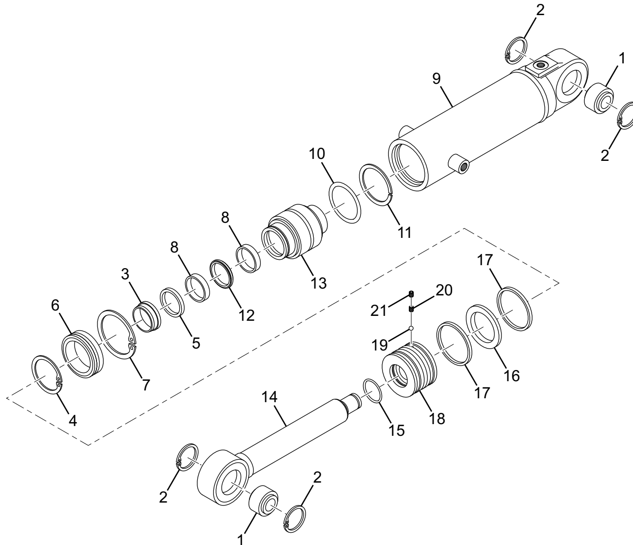
转向油缸 Steering Cylinder (LG853.06.03) (图 /Figure 24)
