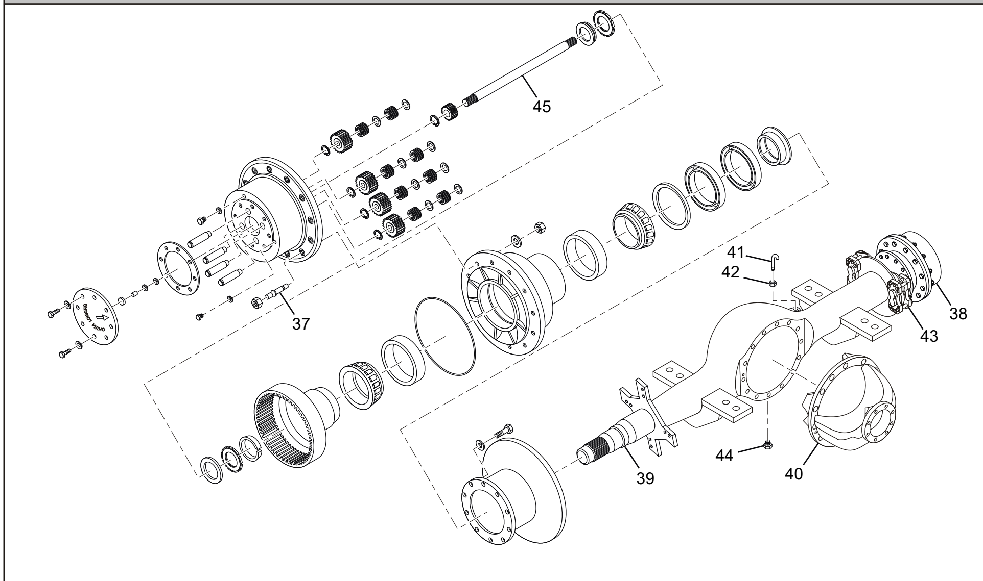
标准 50F 驱动桥 Standard 50F Axle II ( LG50F.04500A 前桥用 LG50F.04800A 后桥用 )( 图 /Figure 18)
