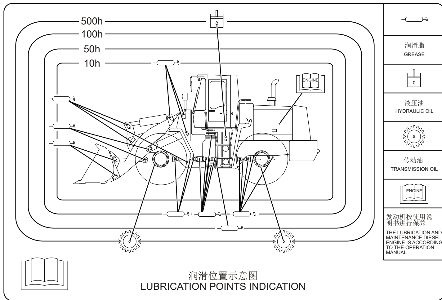
润滑点分布图 GREASING POINTS INDICATION LAYOUT ( 图 /Figure 39)
