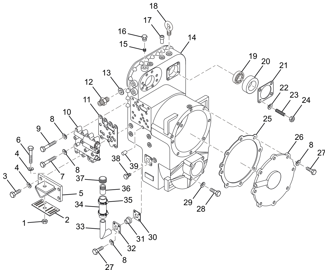
变速箱总成 I Transmission Assembly I (LG853.03.01) ( 图 /Figure 09)
